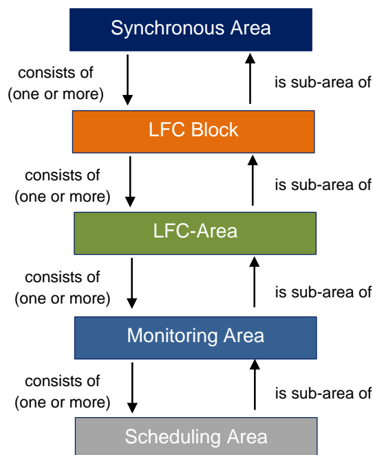
Joonis 1. CE SA sageduse juhtimise struktuur
